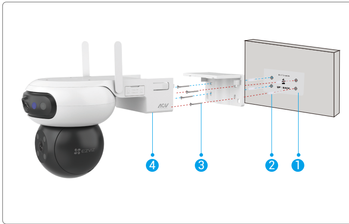
그림 2 벽 장착
